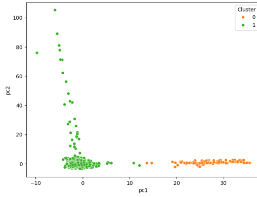
圖 5.2: 未移除 outlier 做 pca+kmeans 的 SMOTEdat
