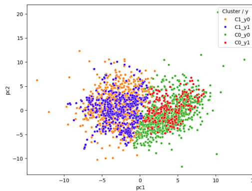
圖 5.5: 移除 outlier 做 pca+kmeans 的 SMOTEdata 含 y
