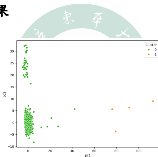
圖 5.1: 未移除 outlier 做 pca+kmeans
