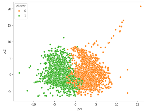
圖 5.4: 移除 outlier 做 pca+kmeans 的 SMOTEdata
