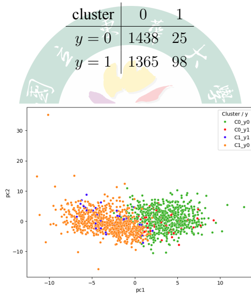
圖 5.3: 移除 outlier 做 pca+kmeans 的原始 data 含 y
